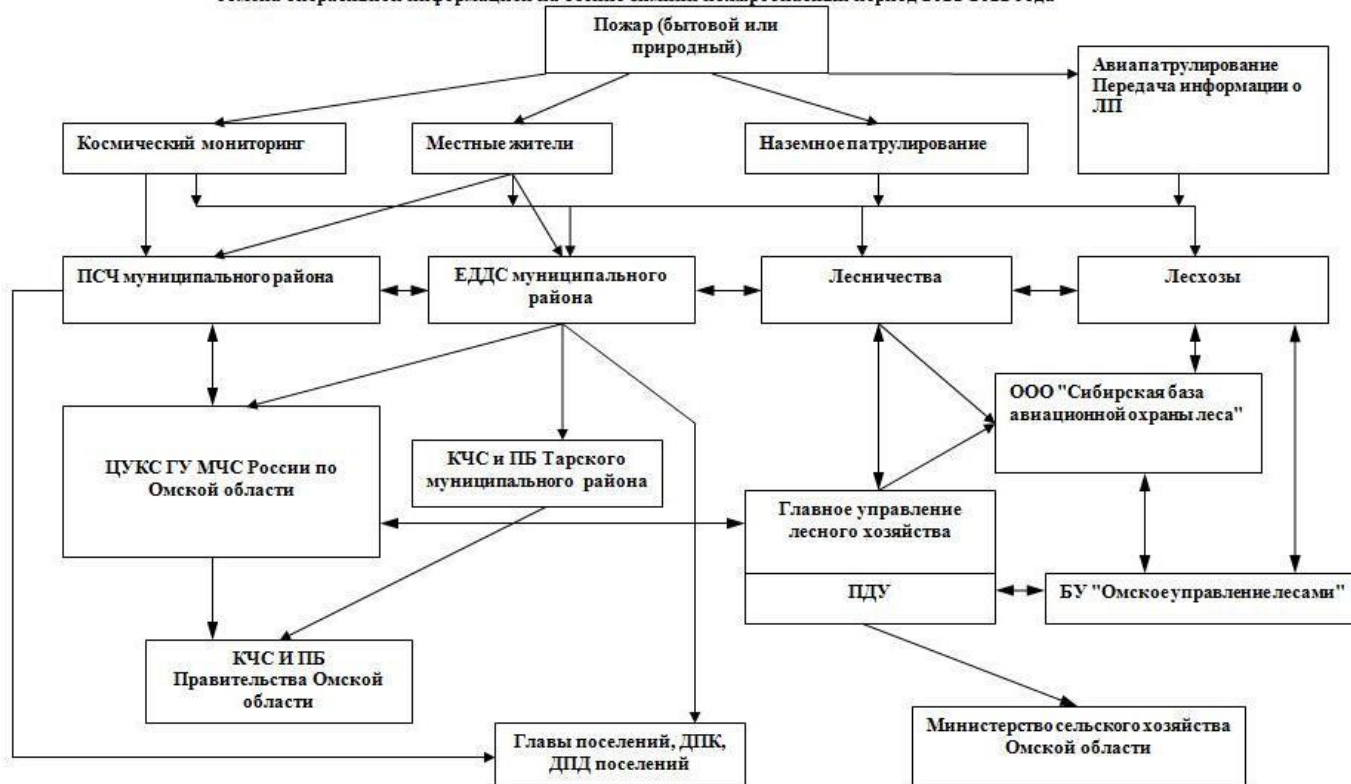
Схема обмена оперативной информацией на осенне-зимний пожароопасный период 2021-2022 года
